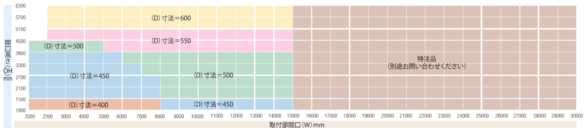
■標準仕様[クリアランス(D)]寸法表
