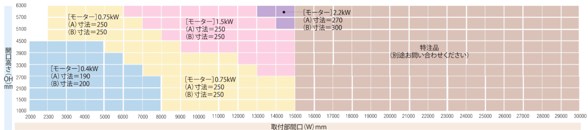
■標準仕様各部寸法表[モーター]容量=(KW) (A)=上部フレーム高さ寸法(B)奥行寸法
